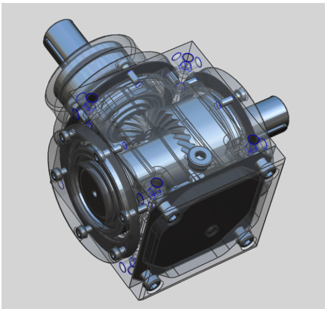
Bild: Kegelradgetriebe mit hermetischem Druckausgleich
